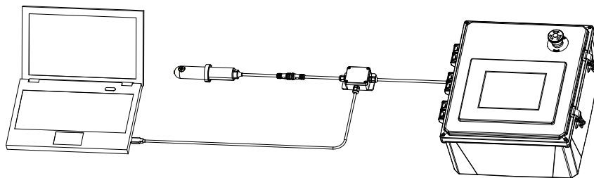
图 4-6 485 适配器连接
